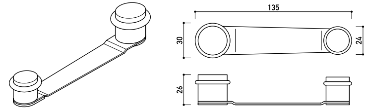
fermaporta elica
