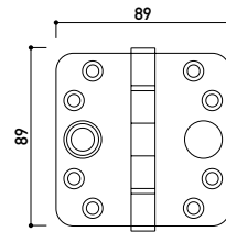
cerniera
