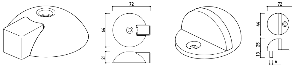
fermaporta tartaruga 2
