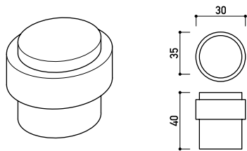
fermaporta fungo
