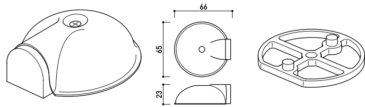
fermaporta tartaruga
