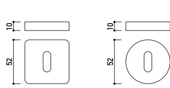
ROSETTE TONDE/QUADRATE
